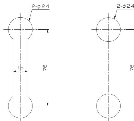
パネルカット図 For panel cut-out
