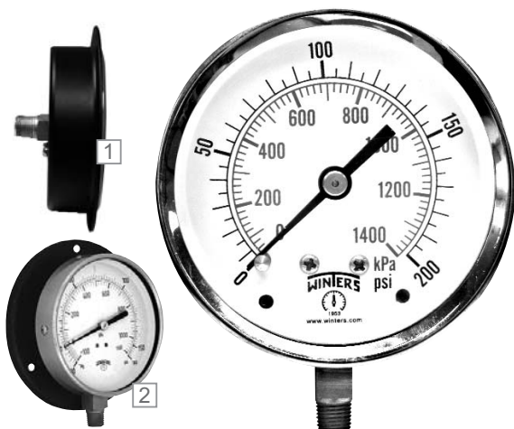
1. Optional Front Flange 2. Optional Back Flange
