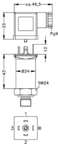
ISO 4400 (IP 65)
